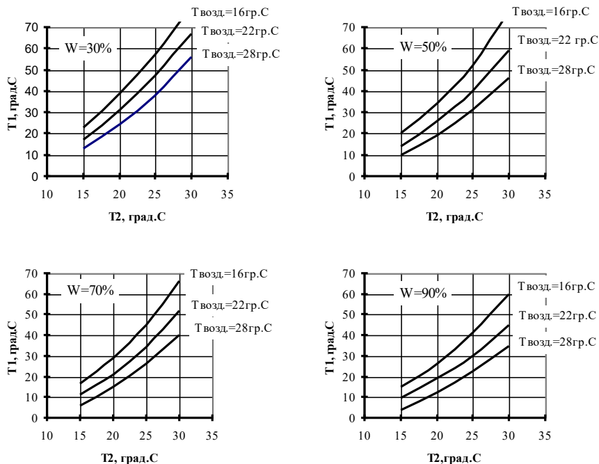
Рис.6. Графики охлаждения при расходе воды 10 м 3 /ч:
